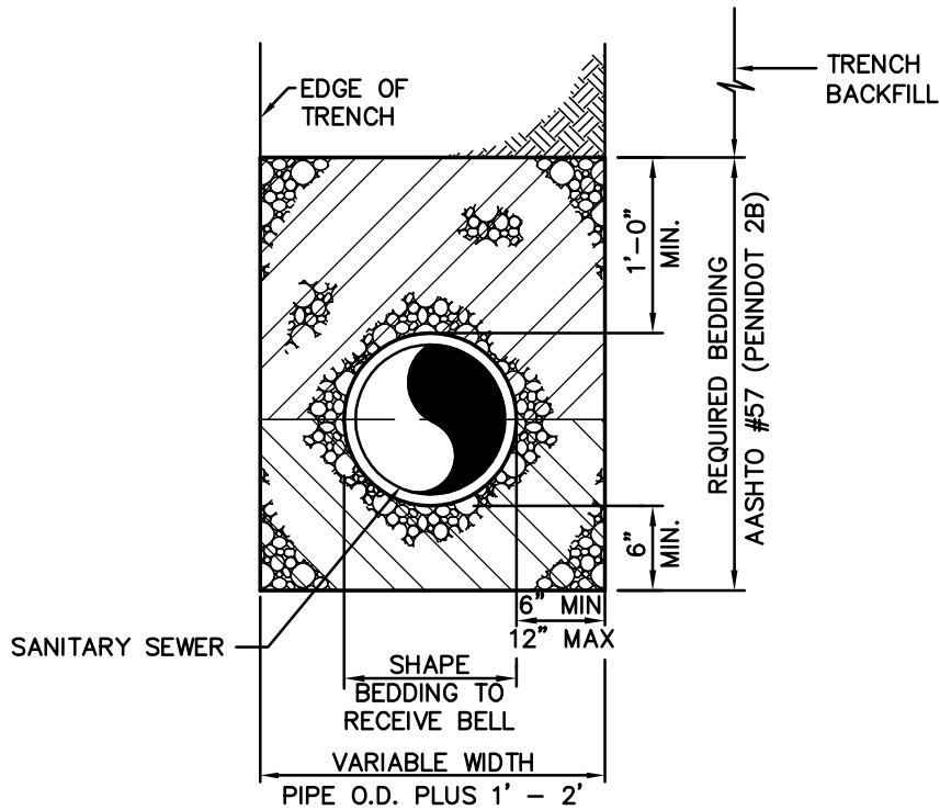
P.V.C. PIPE EMBEDMENT
